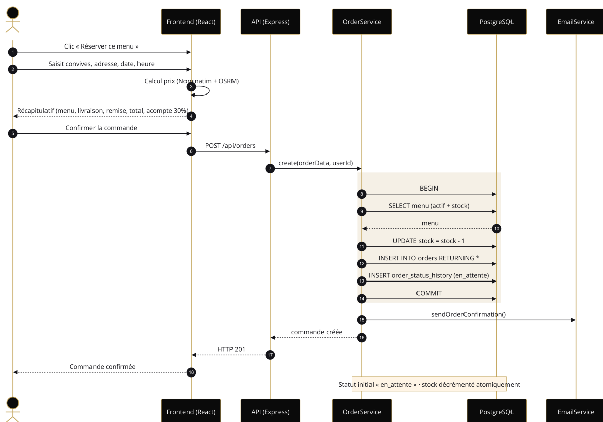
Figure 4 — Diagramme de séquence : commander un menu
